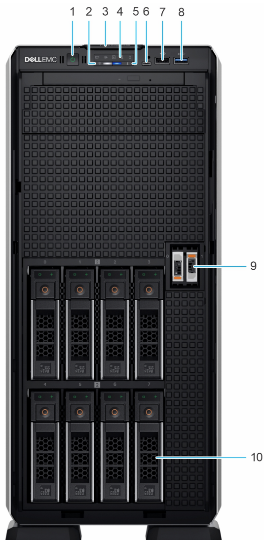
Figura 5. Vista anteriore del sistema con 8 unità da 3,5 pollici (configurazione di upselling)
