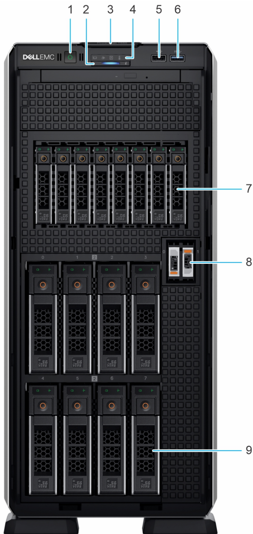
Figura 3. Vista anteriore del sistema con 8 unità da 3,5 pollici + 8 unità da 2,5 pollici
