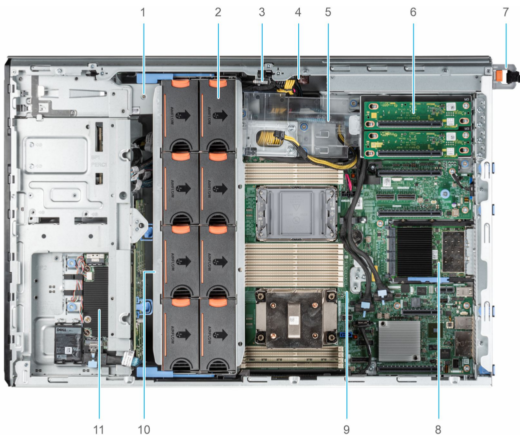
Figura 9. All'interno del sistema per configurazione con 8 unità da 3,5 pollici + 8 unità da 2,5 pollici
