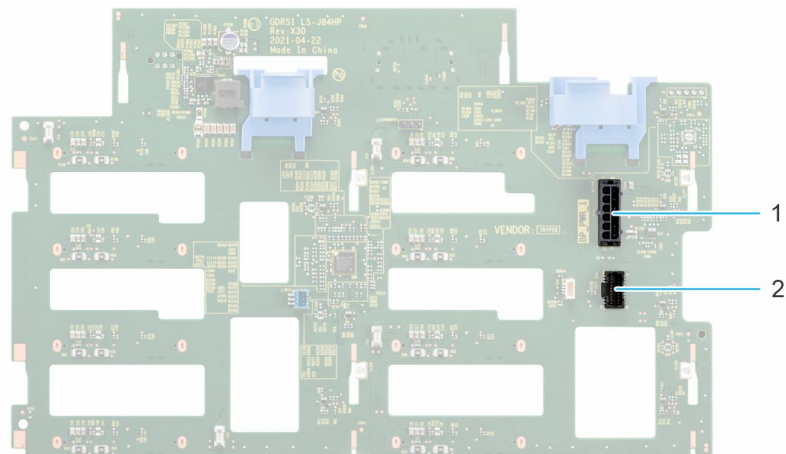
Figura 11. Backplane con unità da 3,5 pollici
